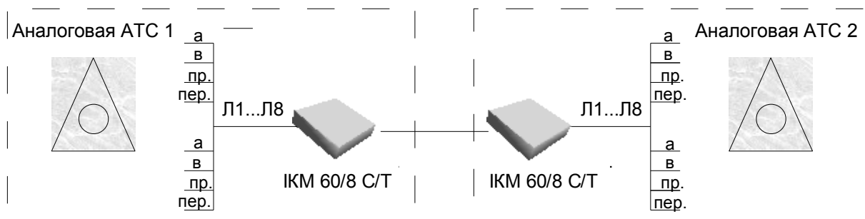
Рисунок 14 - Вариант 3. ИКМ 60/8 С/Т - ИКМ 60/8 С/Т
