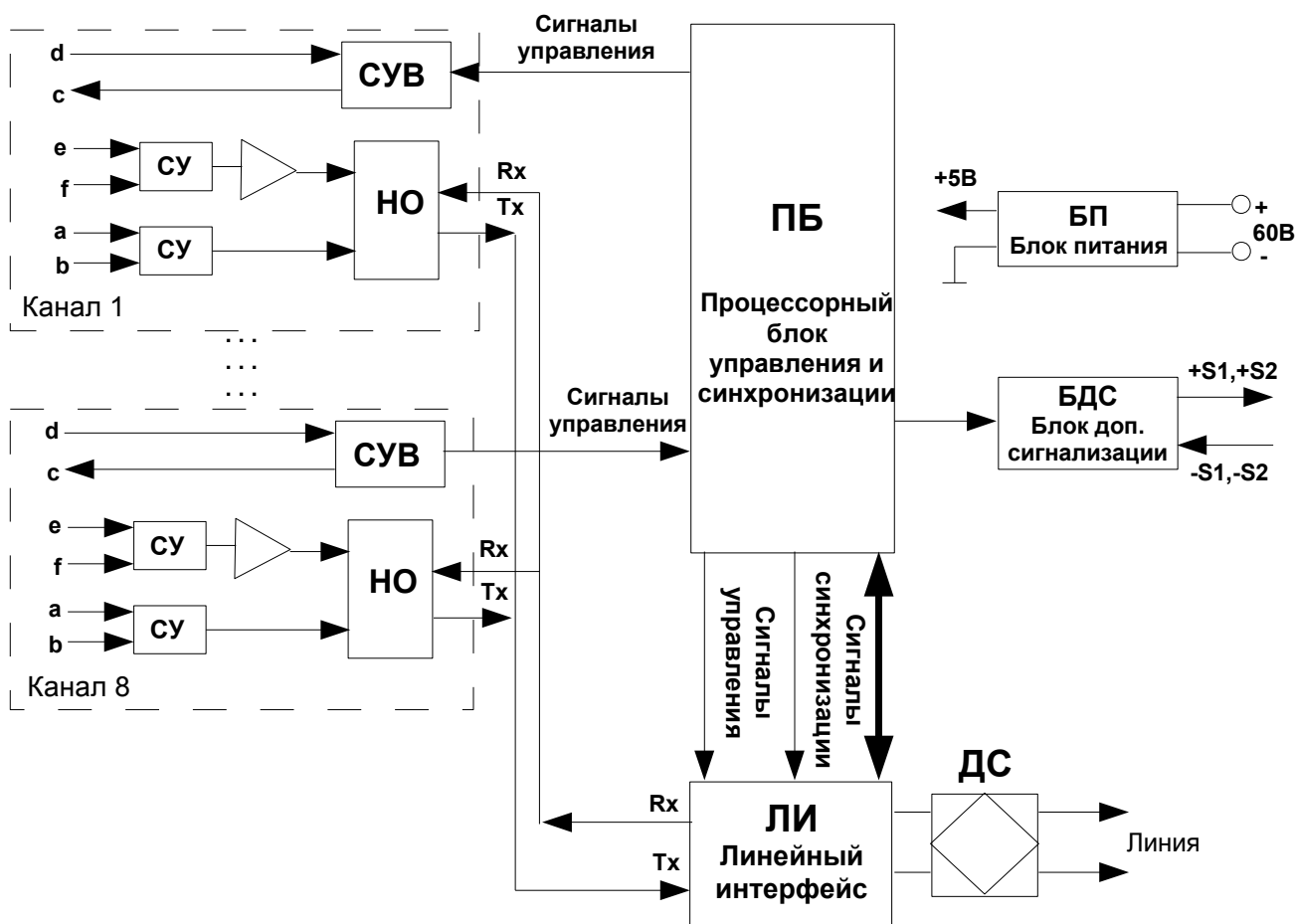
Рисунок 3 - Структурная схема ИКМ 60/8 С/Т
