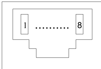
Рисунок 9 - Разъем E1, вид спереди
