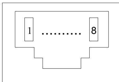
Рисунок 11 - Разъем "Ethernet", вид спереди
